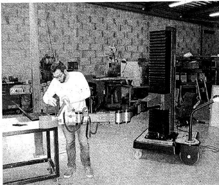
Les techniciens de Neoditech, au Pallet, fabriquent des bras articulés pour répondre aux besoins du secteur industriel.
